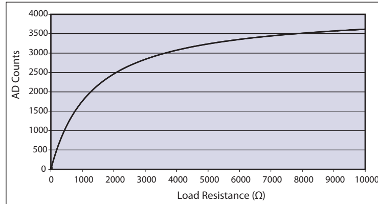
Rheostat Inputs
